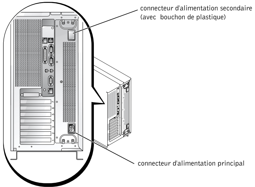
Figure 3-2. Connecteurs d'alimentation
